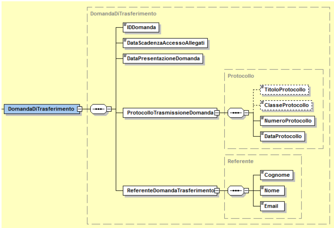
Figura 3: Schema xsd del nodo “DomandaDiTrasferimento”.
