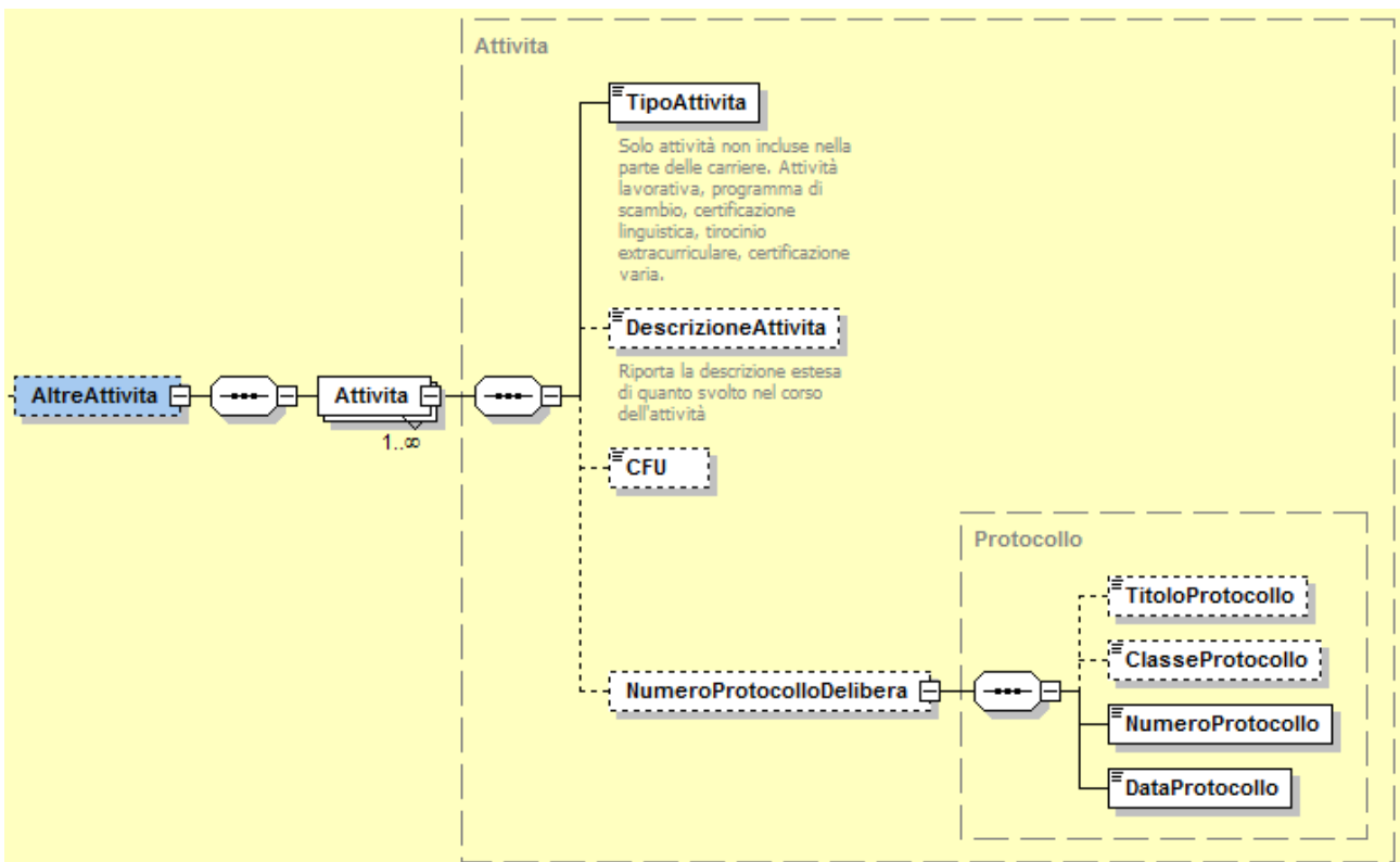
Figura 18: Schema xsd del nodo "AltreAttivita".
