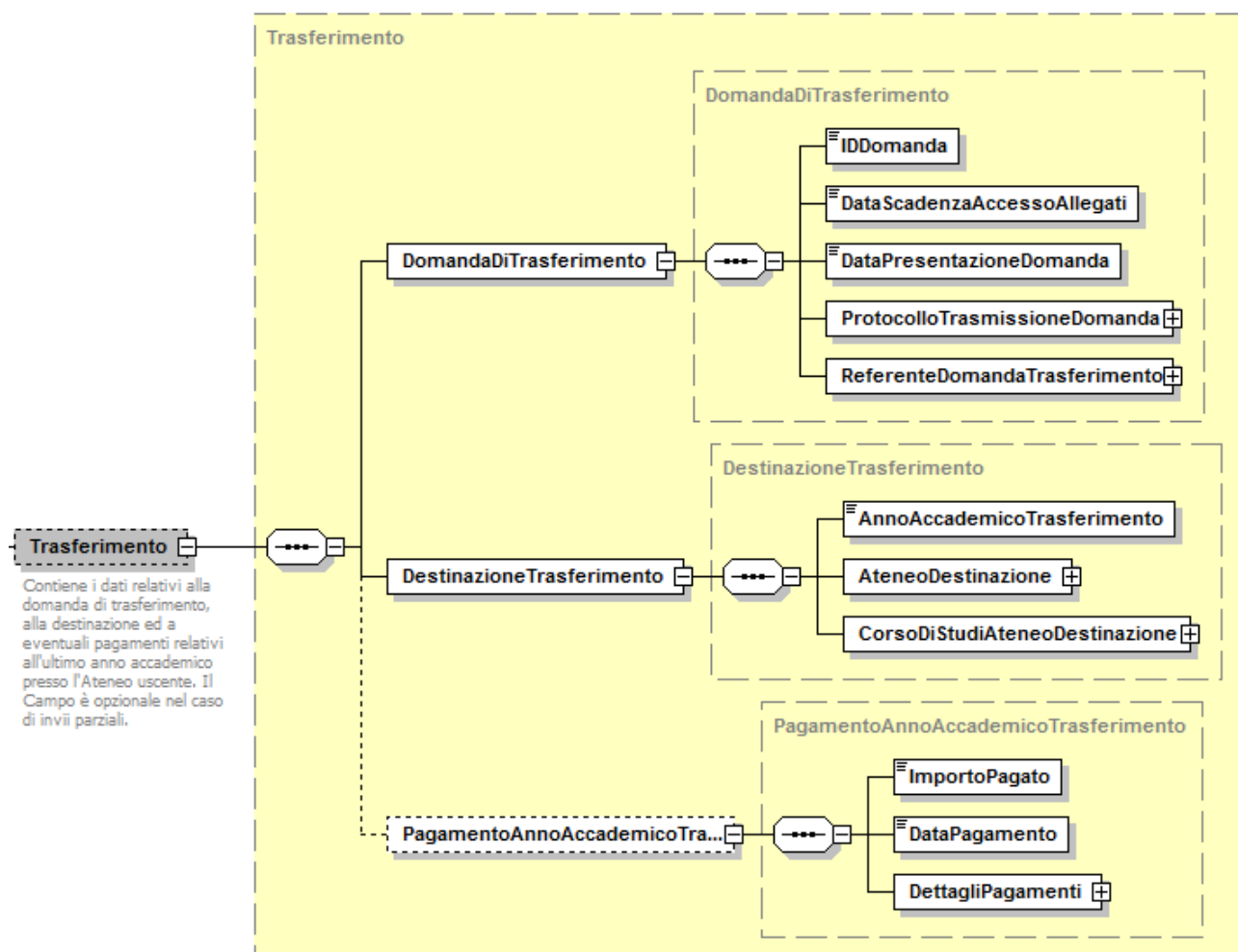
Figura 2: Schema xsd del nodo "Trasferimento".
