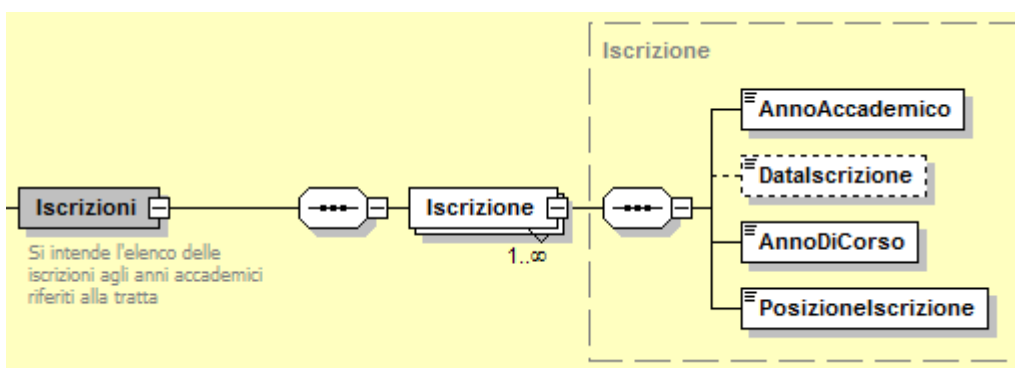
Figura 15: Schema xsd del nodo "Iscrizioni".
