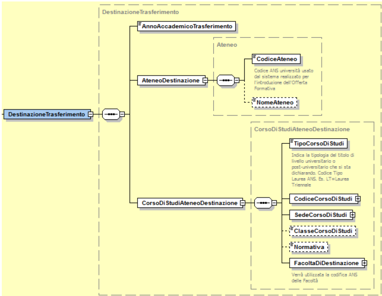
Figura 4: Schema xsd del nodo "DestinazioneTrasferimento".
