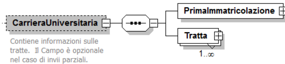
Figura 12: Schema xsd del nodo "Carriera Universitaria".
