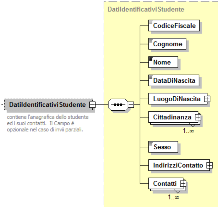
Figura 6: Schema xsd del nodo "DatIdentificativiStudente".
