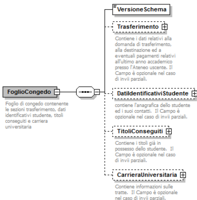
Figura 1: Schema xsd del nodo "FoglioCongedo".
