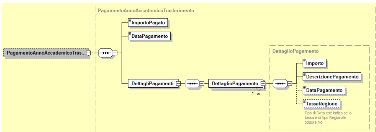
Figura 5: Schema xsd del nodo "PagamentoAnnoAccademicoTrasferimento".
