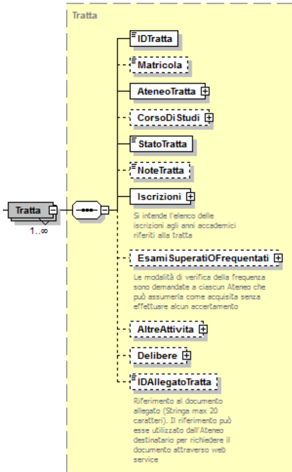
Figura 14: Schema xsd del nodo "Tratta".
